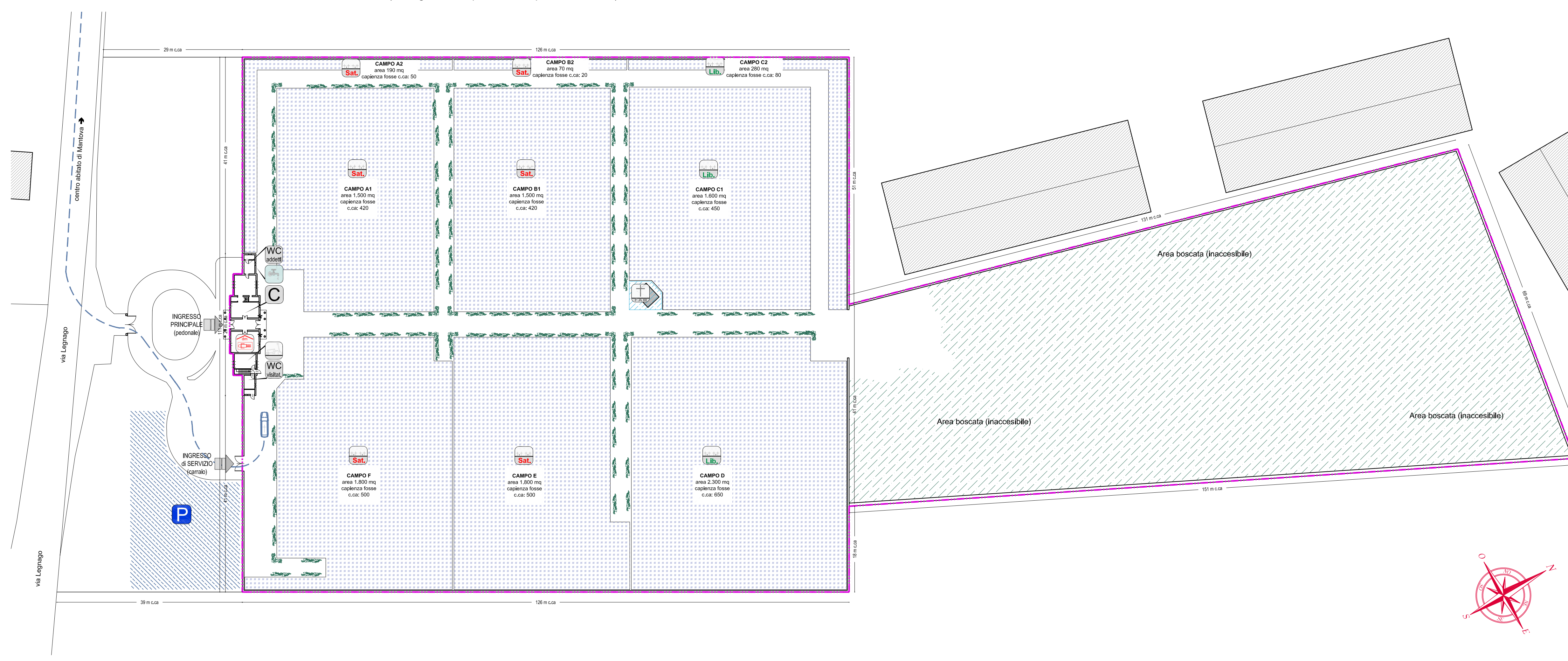
PLANIMETRIA GENERALE DEL CAMPOSANTO . scala 1:500 - (La legenda è riportata su specifica tavola)
