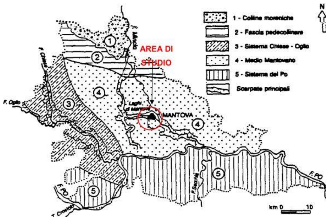
Figura 2.3.2. Unità idrogeologiche della Provincia di Mantova (Baraldi e Zavatti, 1994)
