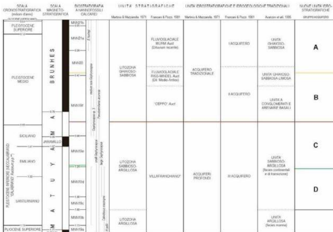
Figura 2.3.3. Schema dei rapporti stratigrafici (Regione Lombardia-Eni, 2002)
