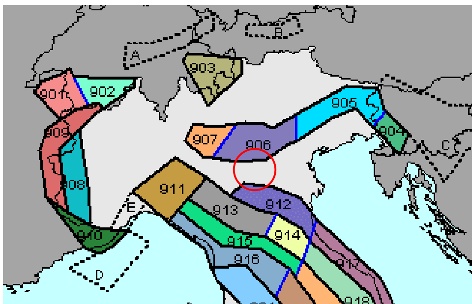
Figura 5.2.2. Zonazione Sismogenetica ZS9
