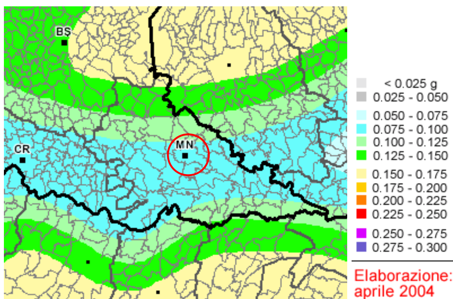
Figura 5.2.3. Nuova mappa di pericolosità sismica
