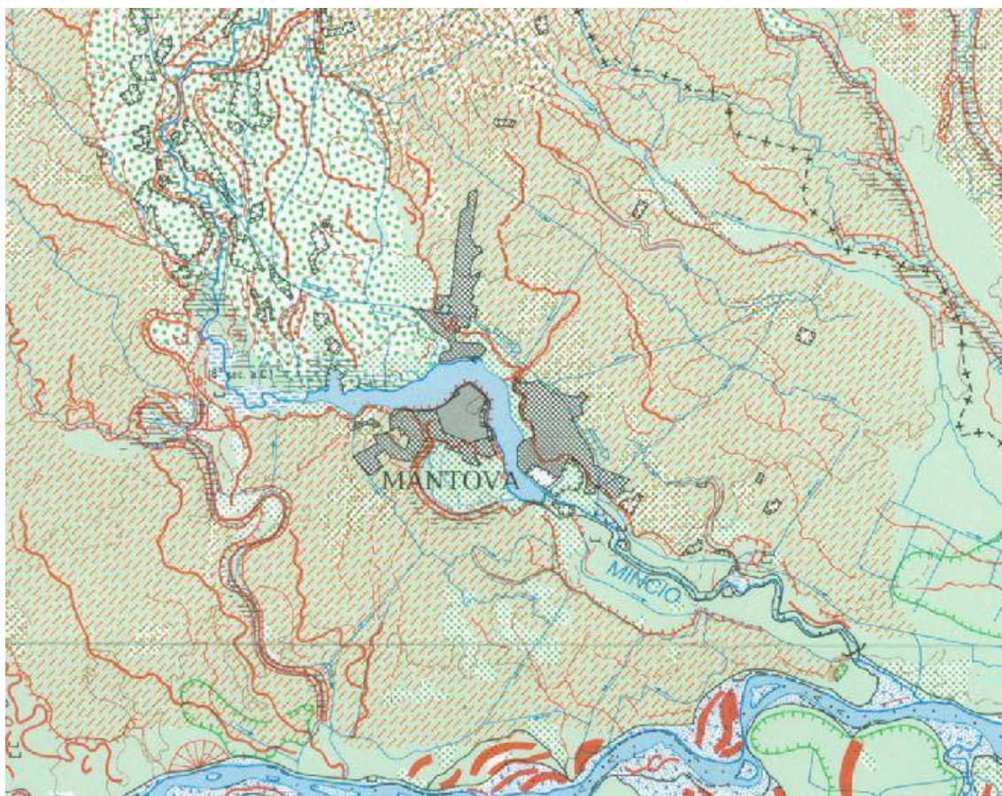
Figura 2.2.1. Carta geomorfologica della Pianura Padana – Ministero dell'Università e della Ricerca Scientifica e Tecnologica. Ed. SELCA 1997
