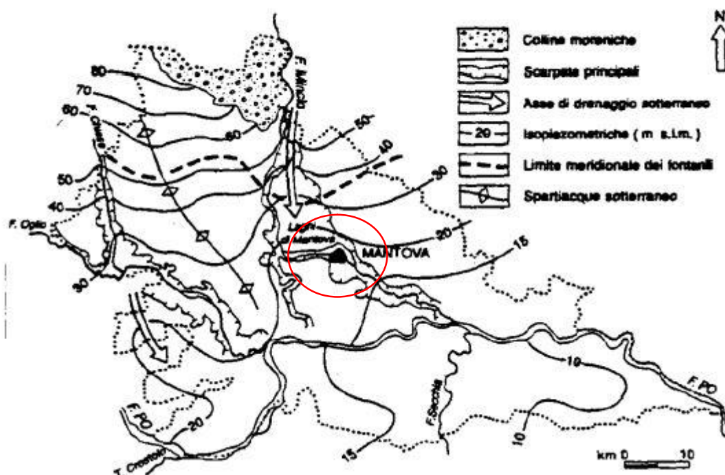
Figura 2.3.4. Morfologia del tetto della falda del primo acquifero (Baraldi e Zavatti, 1994)
