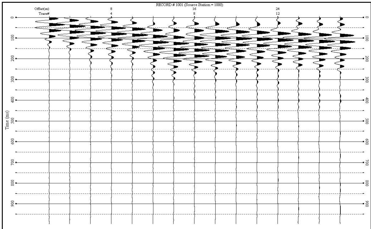
- Sismogramma -
